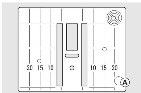
5,5 mm (marquage en mm)
